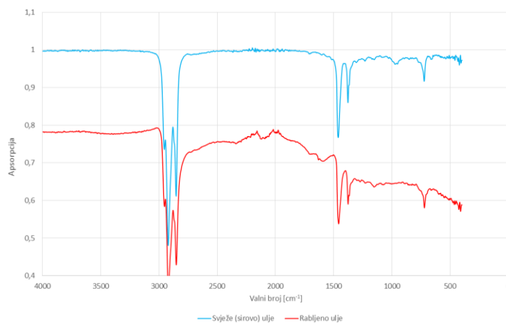
Slika 3.3. Infracrveni transmisijni spektri uzoraka rabljenih ulja
