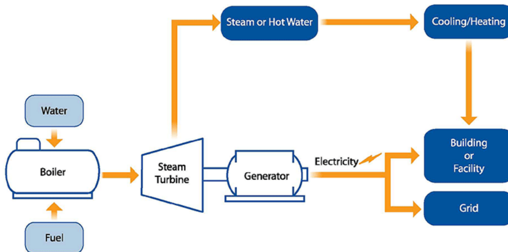
Slika 1.4: Jednostavna shema kogeneracijskog procesa [4]
