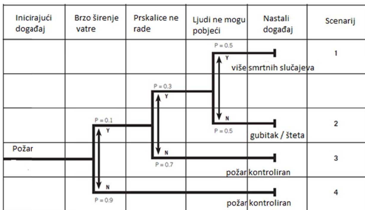
Slika 14. Stablo događaja [21]
