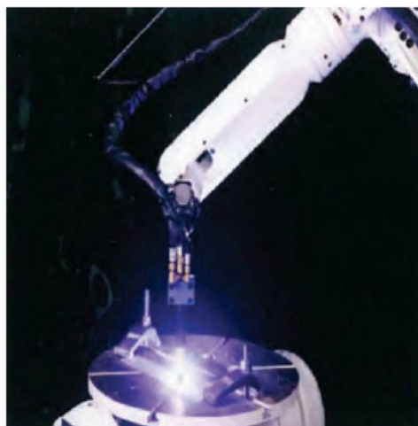
Slika 30. Mehanički kontakti sensor (slika lijevo) i senzor za praćenje napona i struje električnog luka prilikom njihavanja (slika desno) [17]
