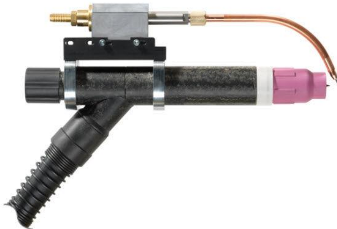
Slika 22. Pištolj za robotizirano TIG zavarivanje s automatskim dodavanjem dodatnog materijala 2 [19]
