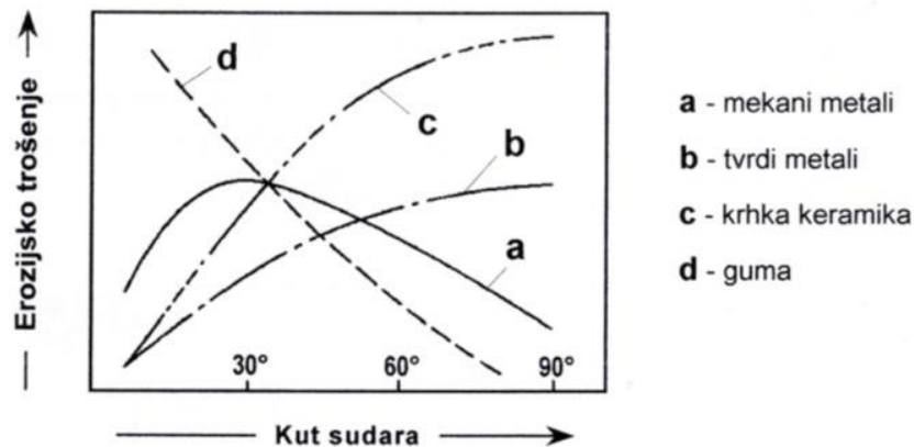
Slika 5.10. Utjecaj kuta udara na erozijsko trošenje krutih čestica [4].
