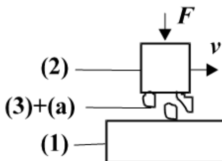
Slika 5.2. Shema tribosustava abrazijskog trošenja; gdje je: (1) - funkcionalni dio, (2) funkcionalni dio, (3) - međusredstvo (mazivo), (a) – abraziv, F – sila, v – brzina [4].
