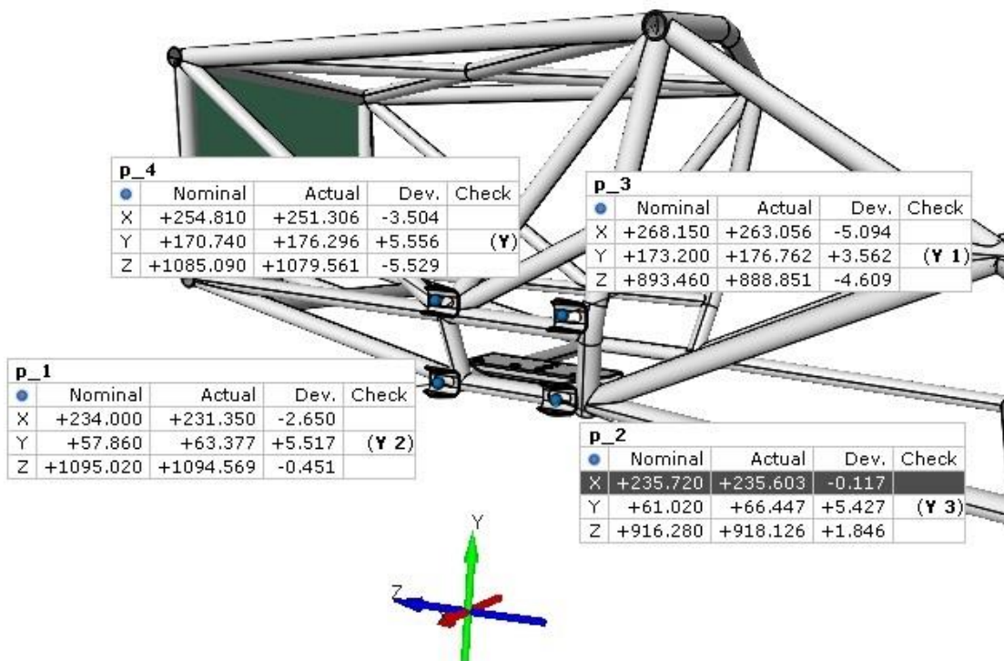
Slika 41. Odstupanja središta prednjih prihвата ramena
