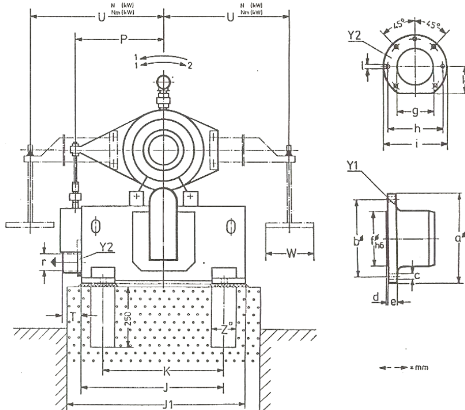
Slika 3.8. Nacrtni prikaz osnovnih mjera kočnice SCHENCK tip D 400 – 1e [5]
