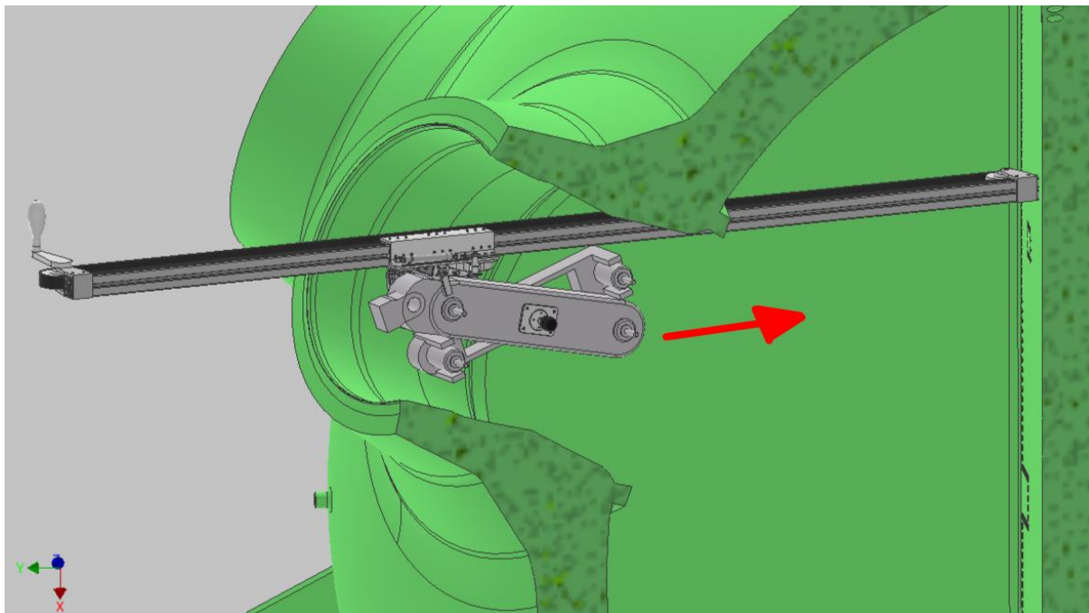
Slika 72. Prolazak kroz otvor parogeneratorsa
