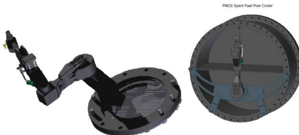
Slika 16. Načini prihвата sustava Spyder na prirubnice
