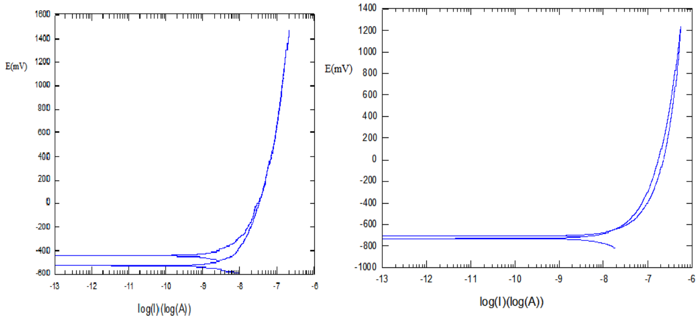
Slika 28. Krivulje cikličkih polarizacija Co-Cr-Mo legure ( 20^\circ\text{C} , 36^\circ\text{C} )
