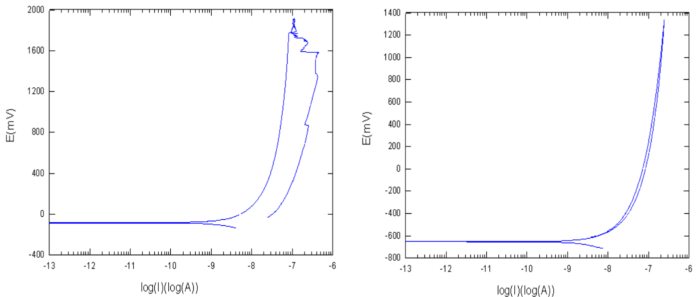
Slika 29. Cikličke polarizacije TiN prevlake ( 36^\circ\text{C} , 20^\circ\text{C} )
