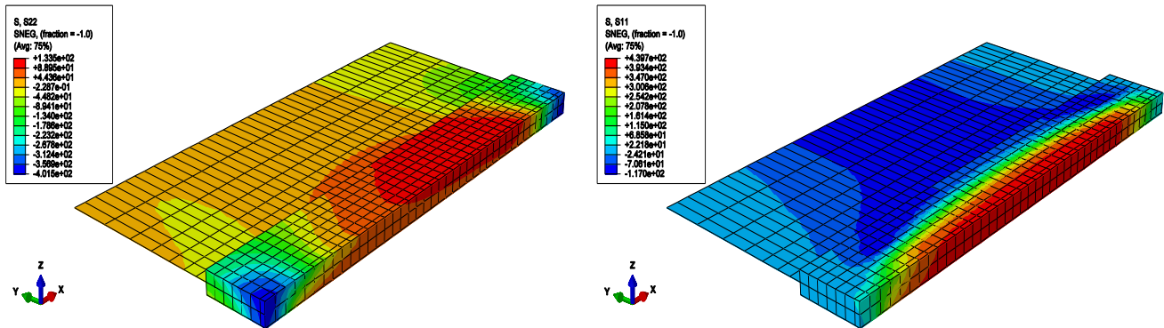
Slika 7.9. Zaostala napreznja kombiniranog modela dobivena metodom rađanja
