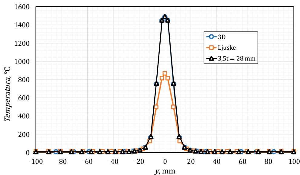
Slika 6.17. Temperaturno polje 3D, ljuskastog i kombiniranog modela
