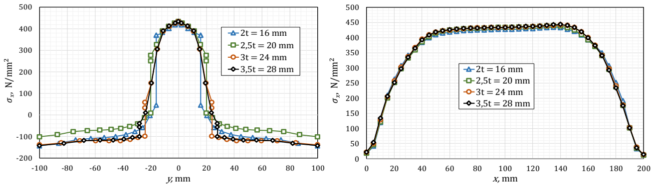
Slika 6.28. Konvergencija uzdužnih naprezanja kombiniranih modela
