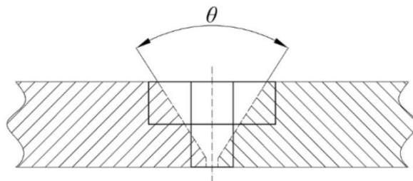
Slika 6.1. Pojednostavljena V priprema zavara
