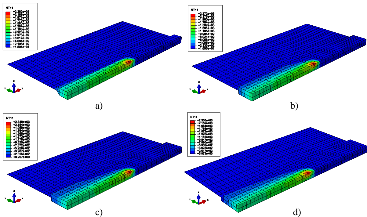
Slika 6.16. Temperaturno polje u 10. sekundi drugog prolaza kombiniranog modela
