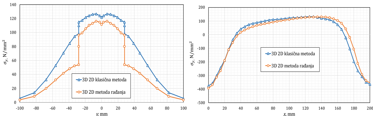
Slika 7.11. Usporedba poprečnih naprezanja kombiniranih modela
