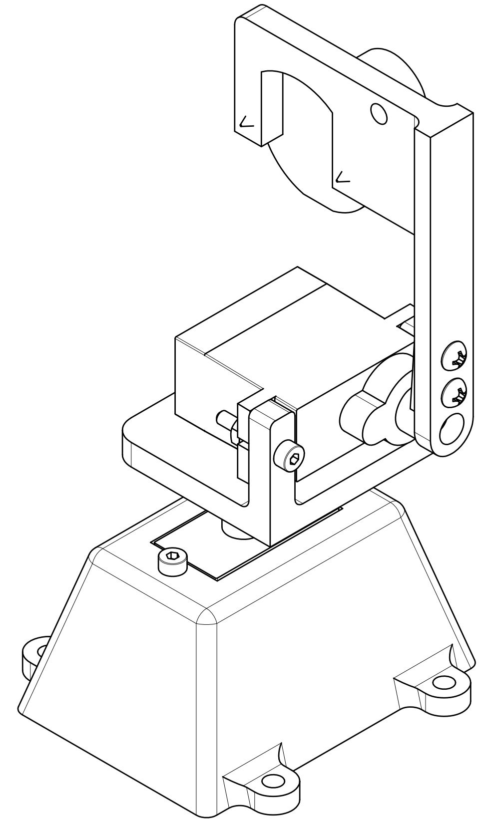
Izometrija M2:1
