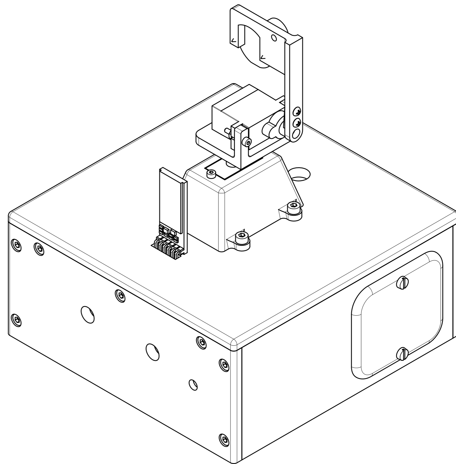
IZOMETRIJA M1:1
