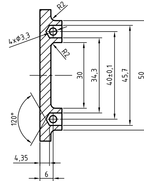
PRESJEK A-A
