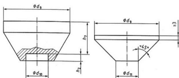
Slika 9. Tlačne ploče [8]
