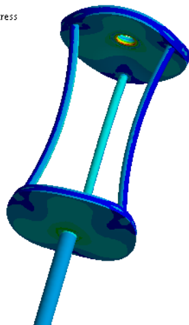
Slika 21. Raspored naprezanja modela sa tri kraka
