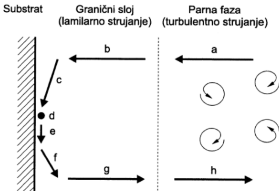
Slika 12. Pojedinačni koraci CVD postupka [22]
