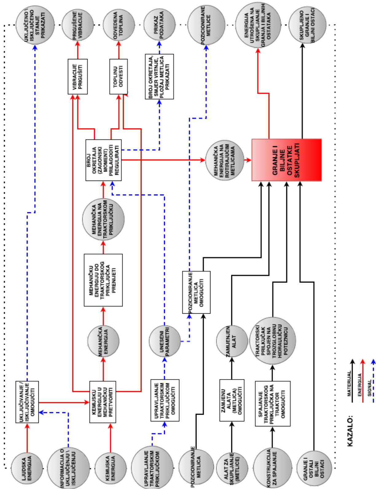
Slika 22. Funkcijska dekompozicija
