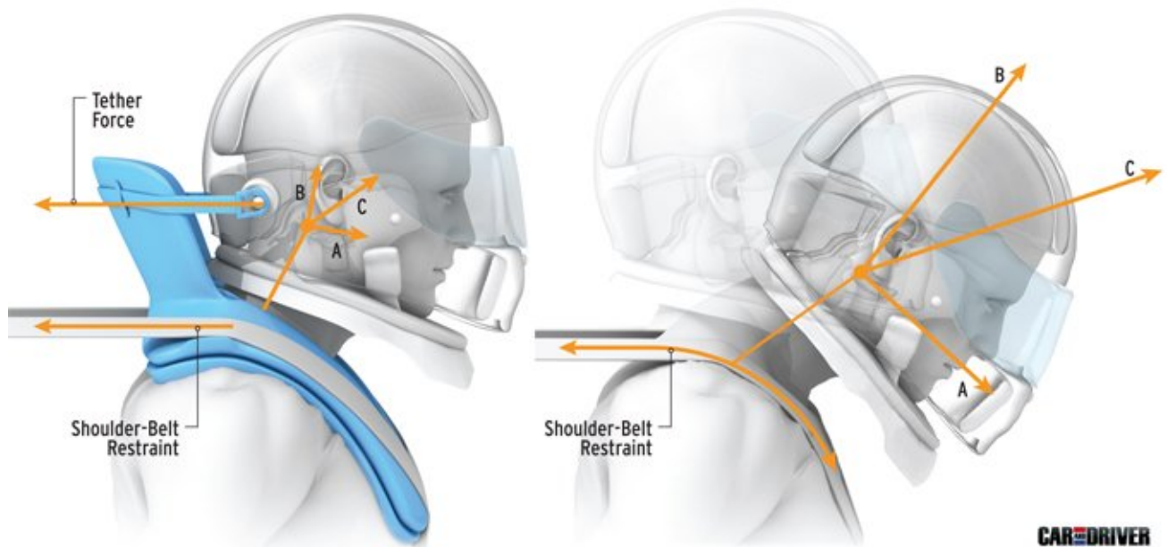
Slika 7. Funkcija HANS uređaja [2]
