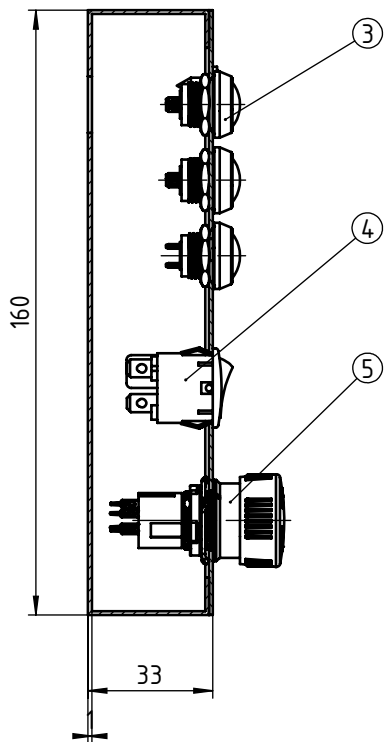
Presjek A-A
