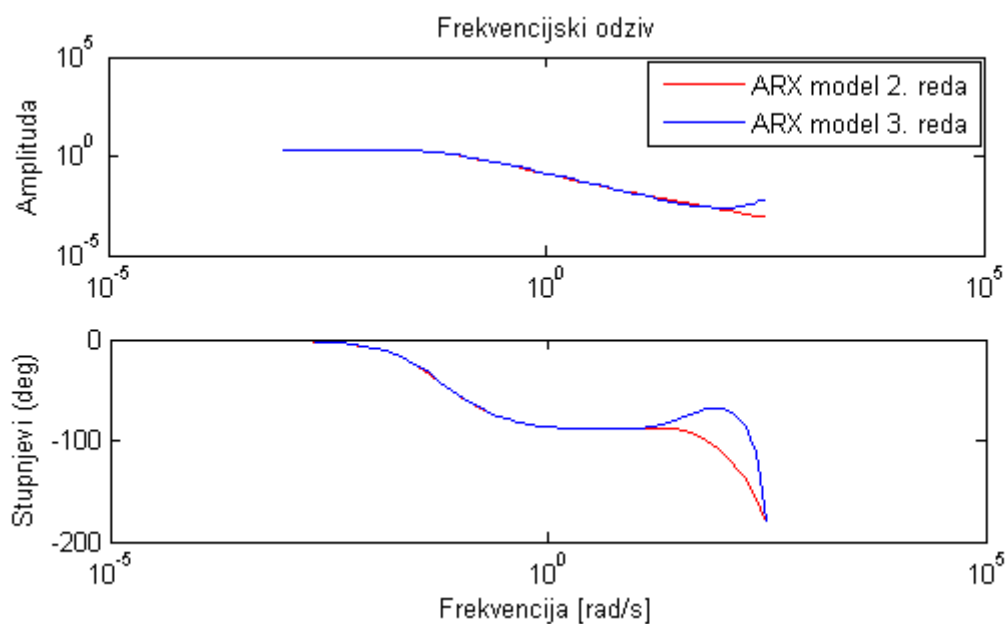
Slika 50. Frekvencijski odziv
