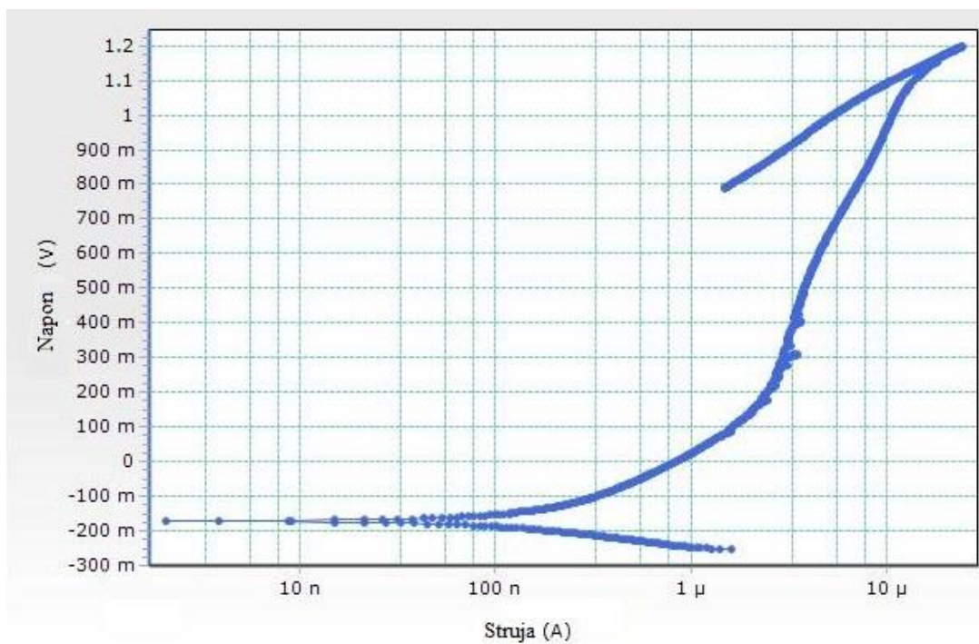
Slika 44. Dijagram cikličke polarizacije za uzorak AISI 316
