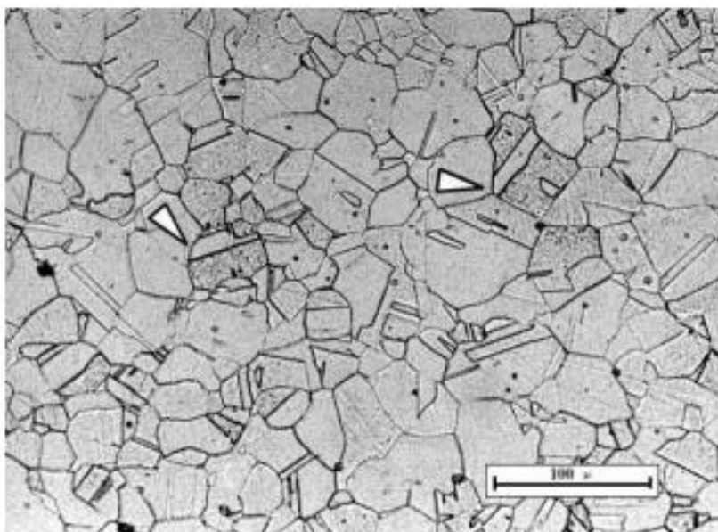
Slika 18. Mikrostruktura austenitnog nehrđajućeg čelika [10]
