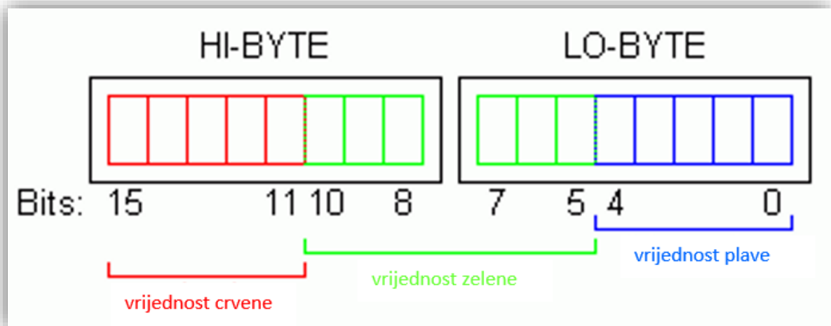
Slika 39. RGB565 [7]
