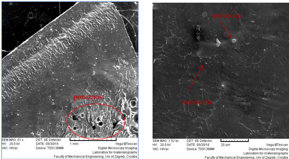
Slika 17 a) uzorak bez ojačanja i b) uzorak bez ojačanja pri većem povećanju
