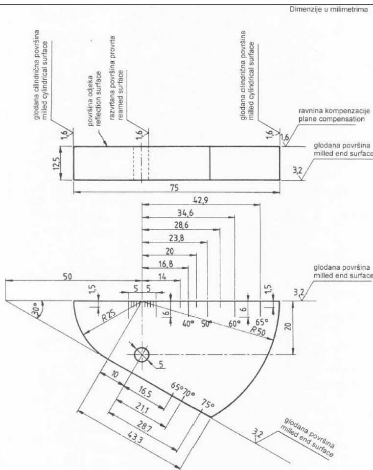
Slika 9. Dimenzije radnog etalona br.2 [8]
