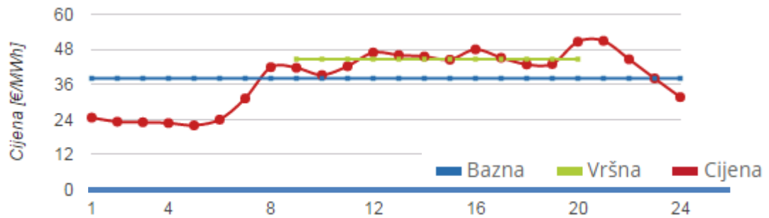
Slika 14. Dnevna krivulja cijena električne energije
