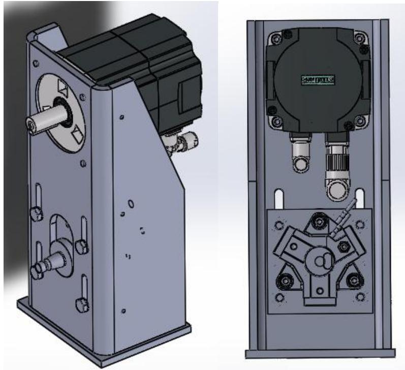
Slika 21. Spoj pumpe i elektromotora na nosač
