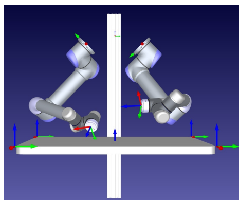
Slika 52: Slika orijentacije baze robota za 135 stupnjeva
