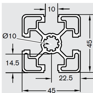
Slika 30: Profil 45x45
