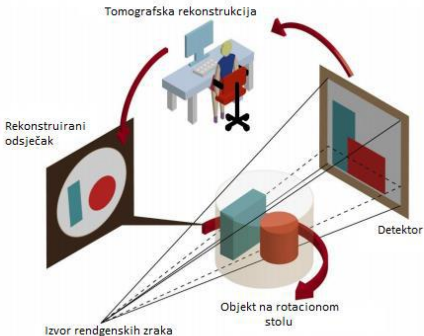
Slika 3. Shema konusnog skenera [1]
