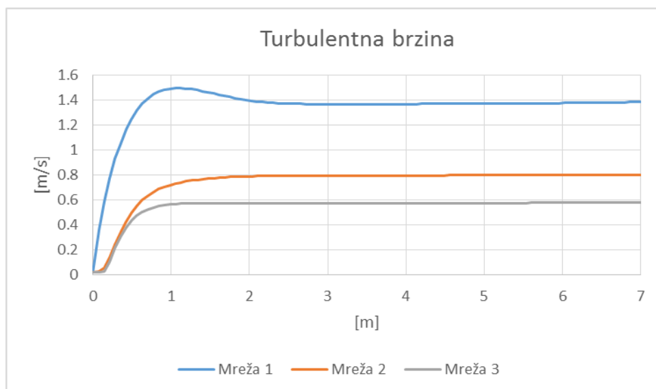
Slika 18. Turbulentna brzina
