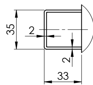
DETALJ B (1 : 2)
