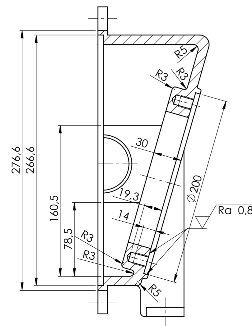
PRESJEK A-A
