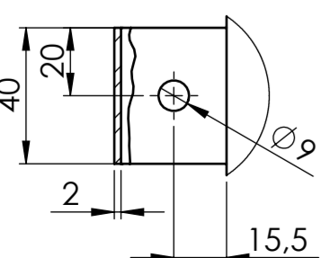
DETALJ A (1 : 2)
