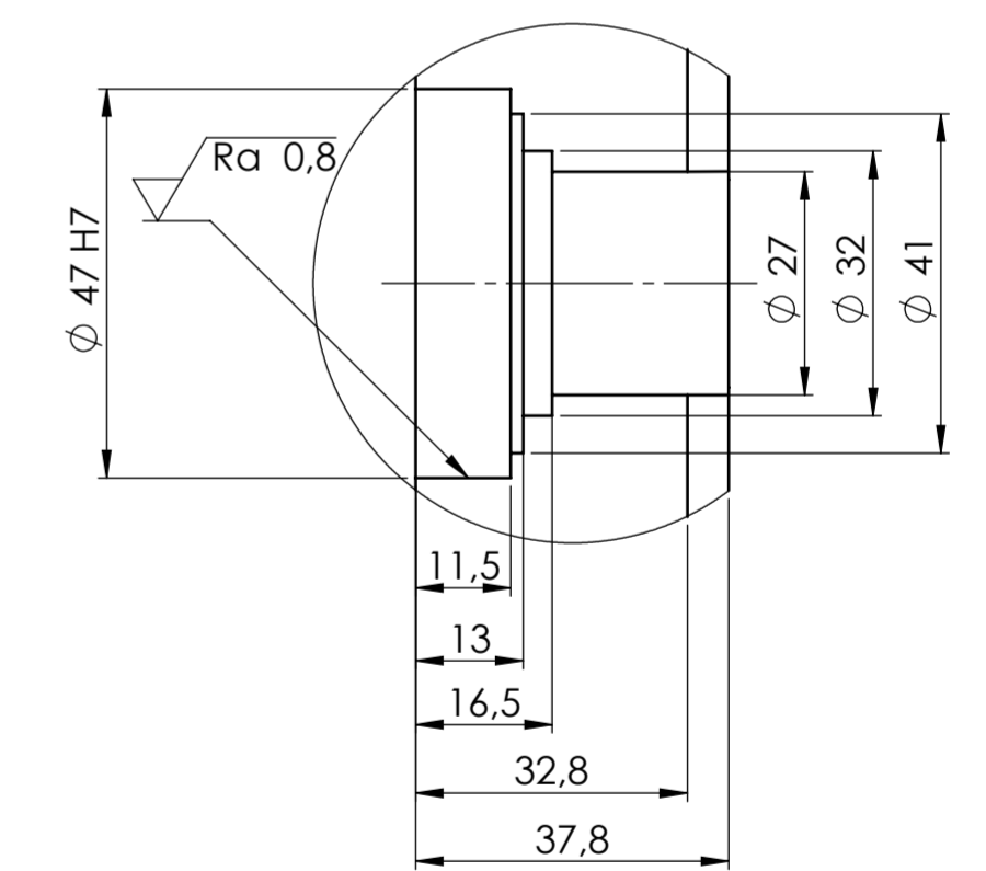
DETALJ D (1 : 1)
