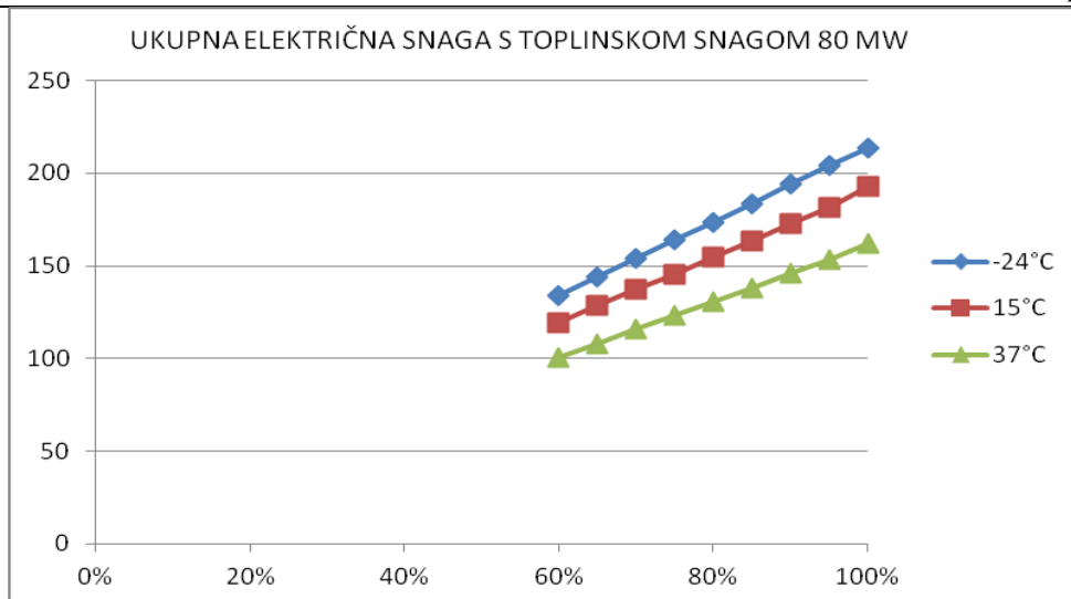
Slika 60. Ukupna električna snaga s toplinskom snagom 80 MW
