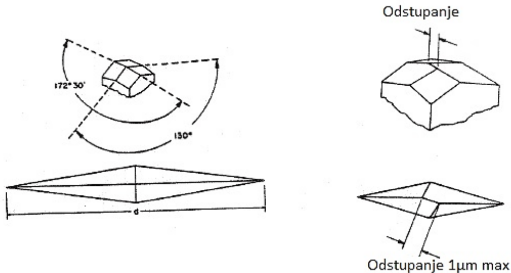
Slika 29. Knoopov indentor i otisak [19]
