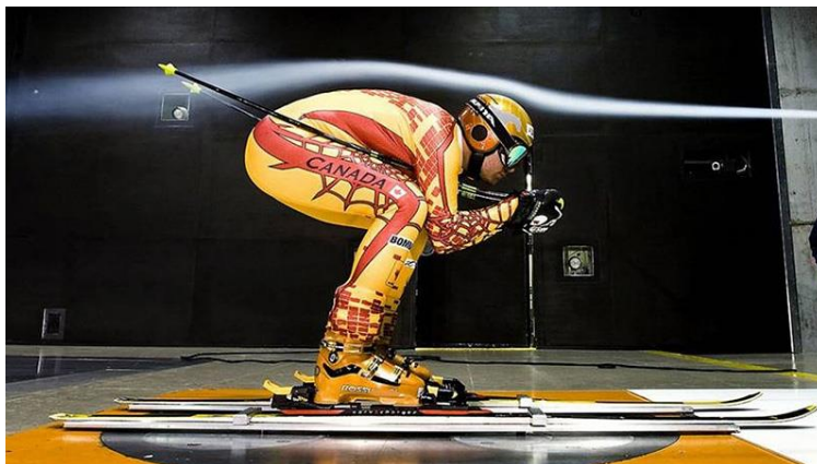
Slika 5. Ispitivanje aerodinamičnosti skijaša [16]
