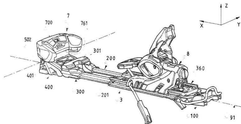
Slika 50. Patent US20120104707A1 – Sigurnosni vez za turno skijanje [42]
