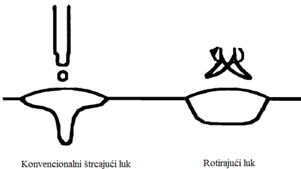
Slika 9. Shematski prikaz prijenosa metala štrcajućim i rotirajućim lukom [8]
