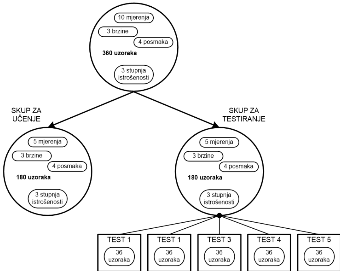
Slika 12. Razvrstavanje podataka u skupove za učenje i testiranje
