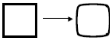
Slika 6. Radijalna distorzija
