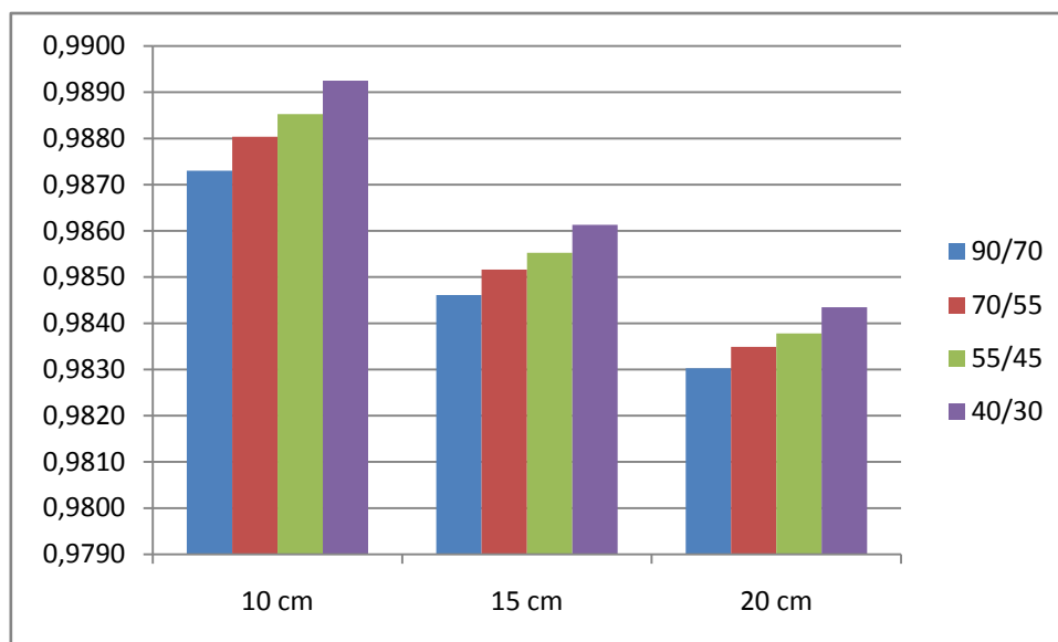
Dijagram 4.4 Ovisnost učinkovitosti kotla o debljini izolacije
