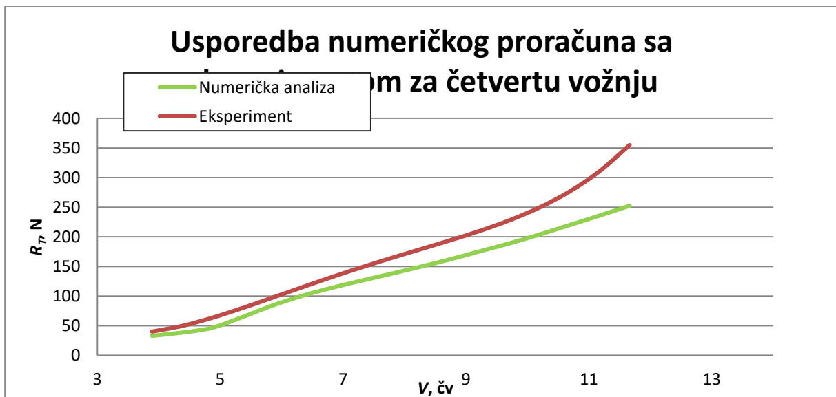
Slika 55. Usporedba numeričkog proračuna s eksperimentom (ovisnost sile otpora i srednje vrijednosti brzine brodicikla u četvrtoj vožnji)
