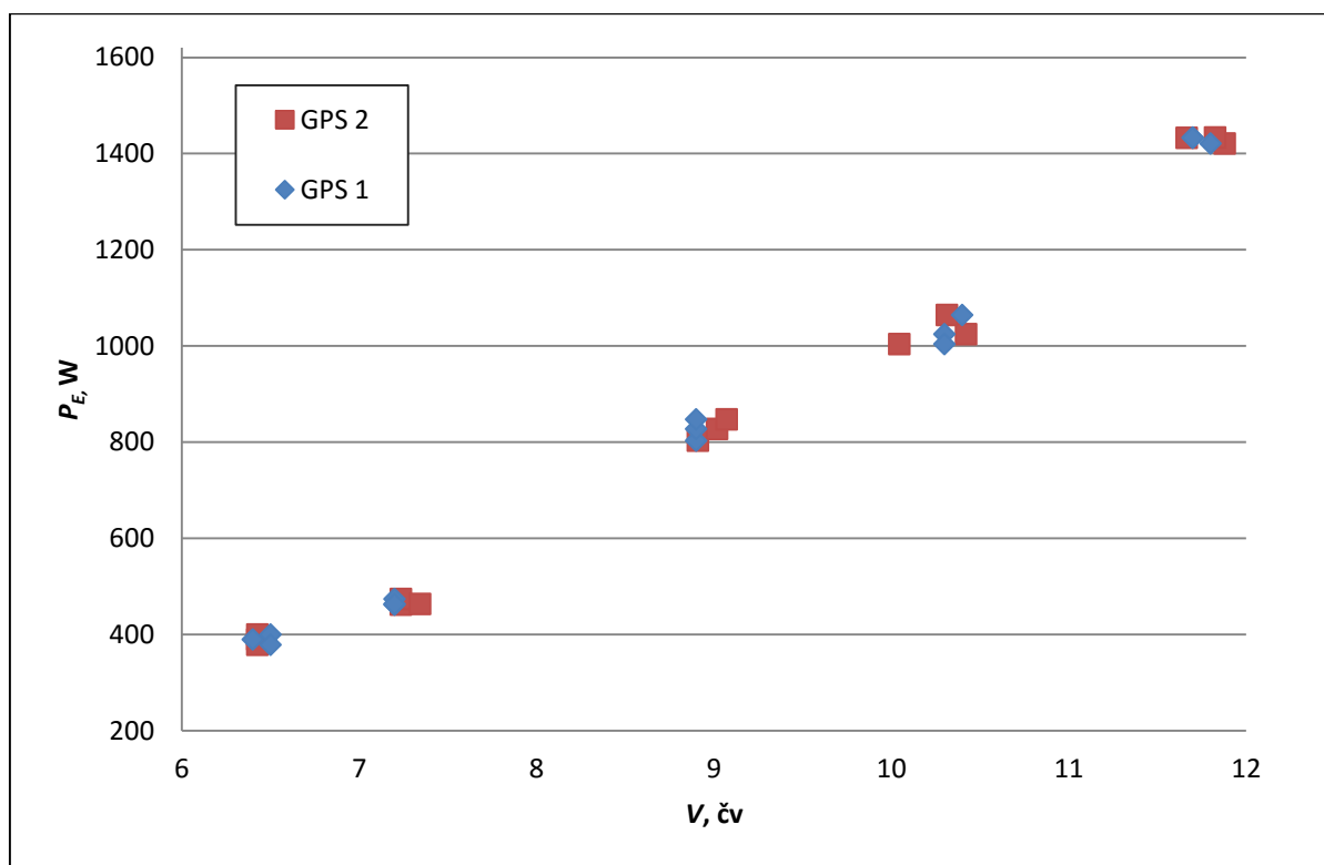
Slika 32. Ovisnost snage i brzine brodocikla u prvoj vožnji
