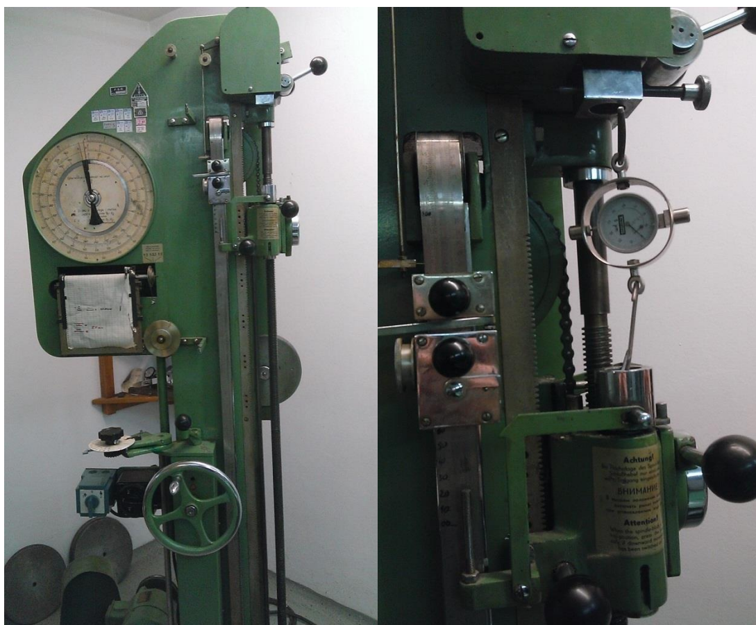
Slika 12. Baždarenje dinamometra
