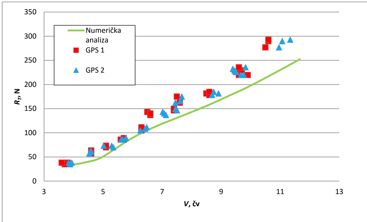
Slika 54. Usporedba numeričkog proračuna s eksperimentom (ovisnost sile otpora i brzine brodicikla u četvrtoj vožnji)
