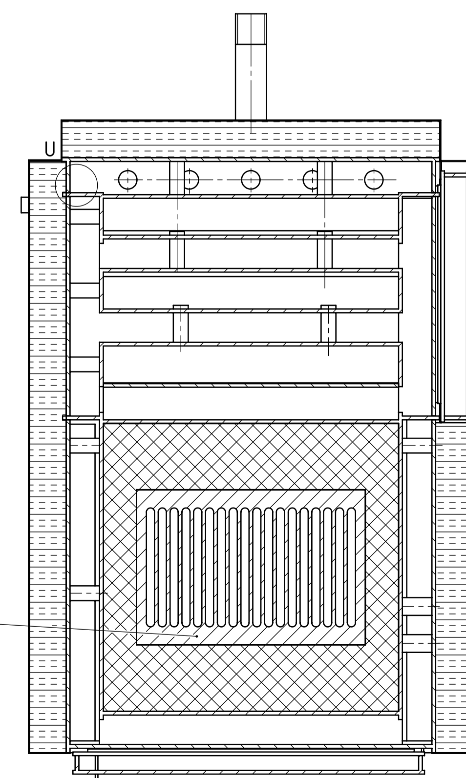
PRESJEK C-C
