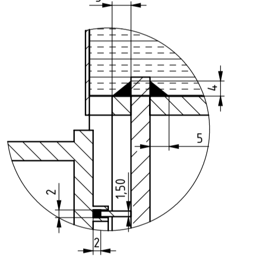
DETALJ T M1 : 1
