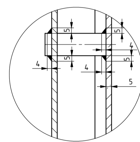
DETALJ Z M1 : 2
