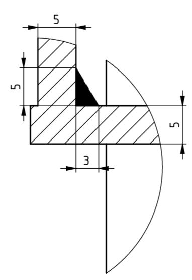
DETALJ V M 2 : 1
