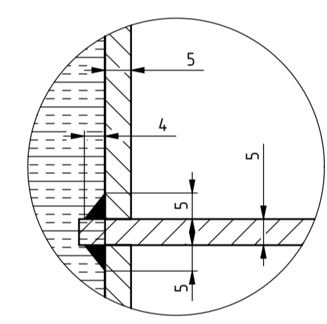
DETALJ U M1 : 1
