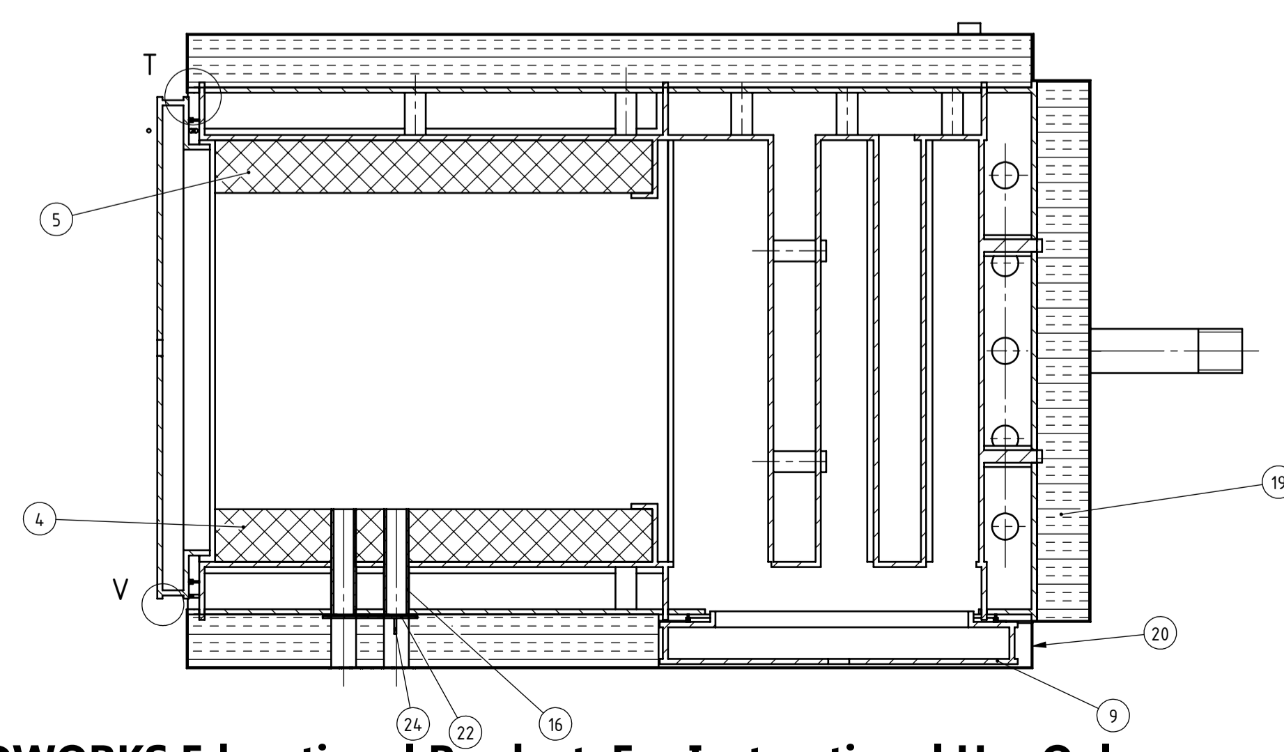
PRESJEK B-B
