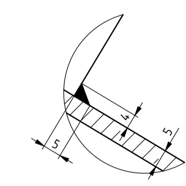
DETALJ Q M1 : 1
