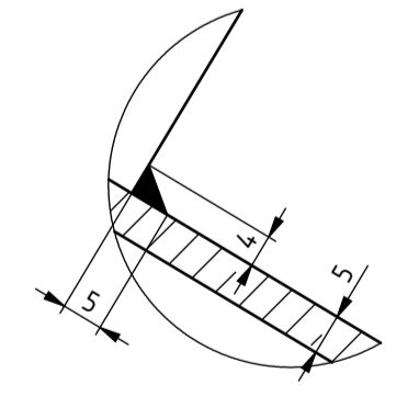
DETALJ Q M1 : 1
