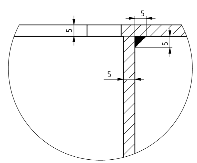
DETALJ Z M 1 : 1
