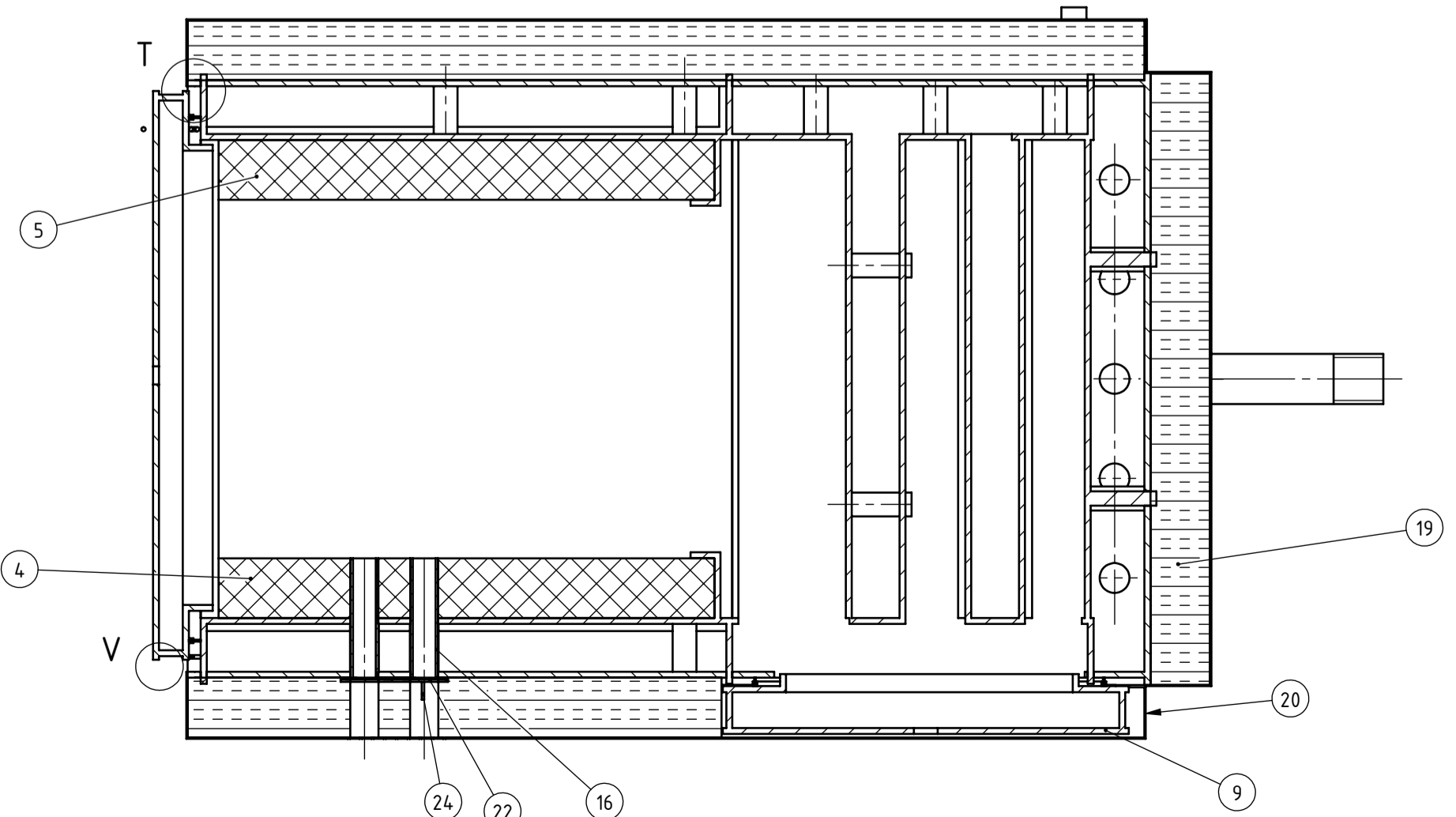
PRESJEK B-B
