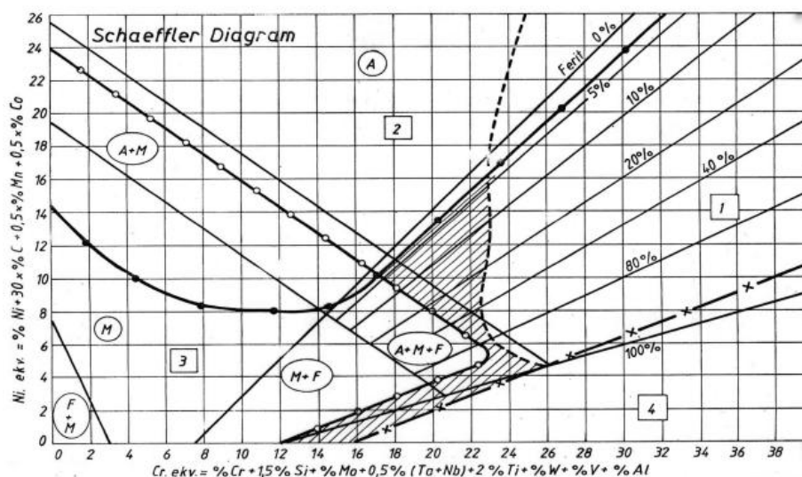
Slika 6. Schaefflerov dijagram [13]
