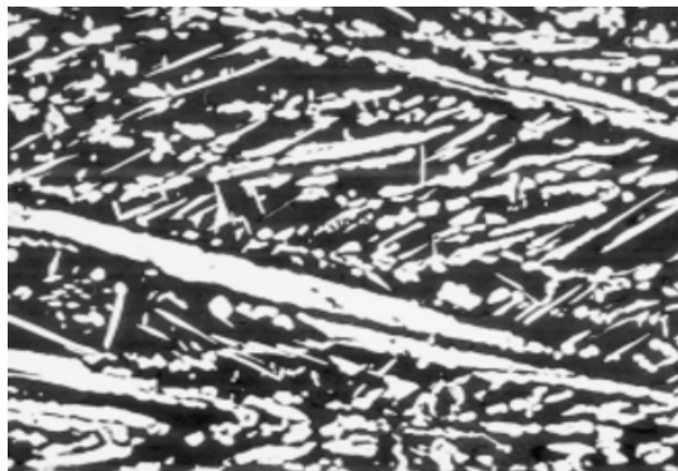
Slika 18. Martenzitna mikrostruktura [30]
