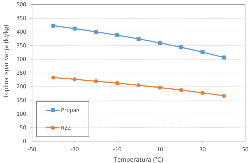
Slika 2 Toplina isparivanja propana i radne tvari R-22
