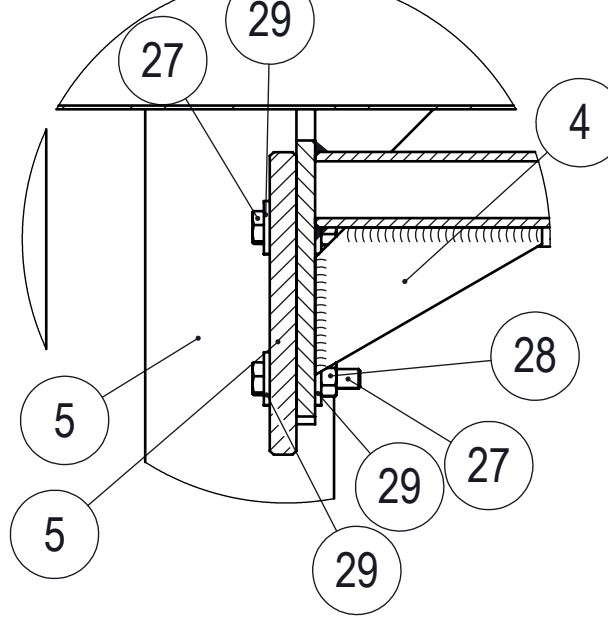
DETALJ H M 1:2
