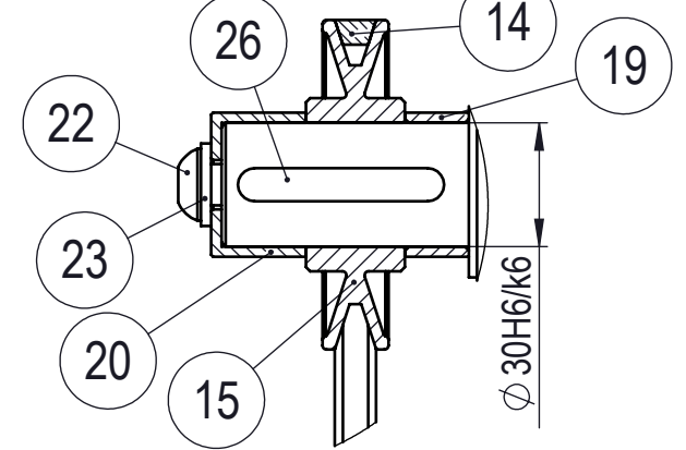
DETALJ E M 1:2
