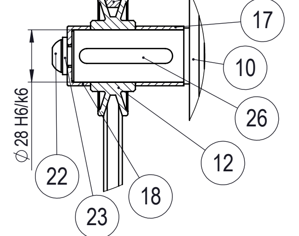
DETALJ E M 1:2
