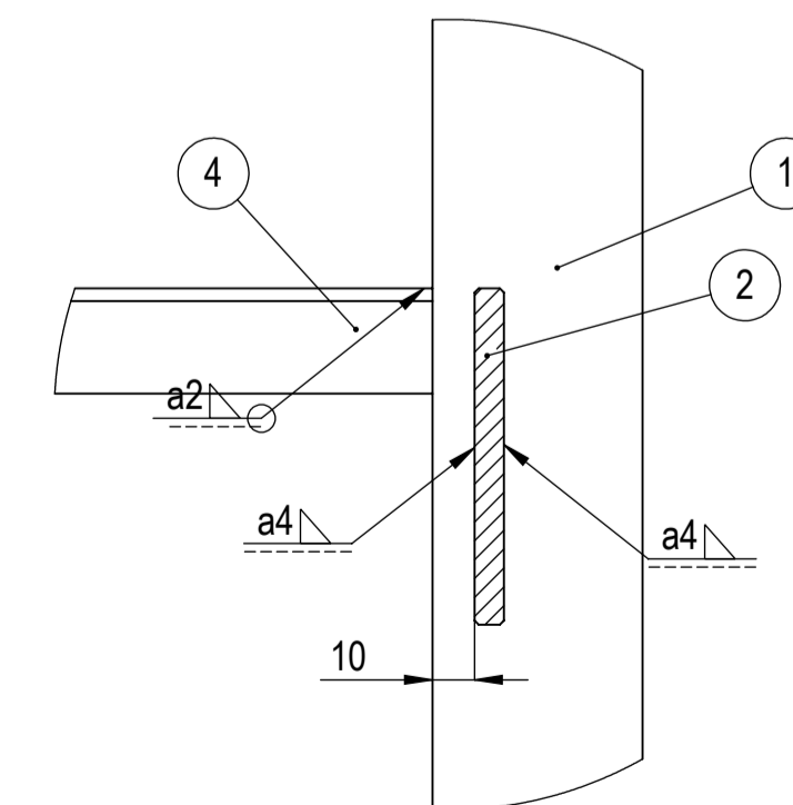
DETALJ K M 1:2
