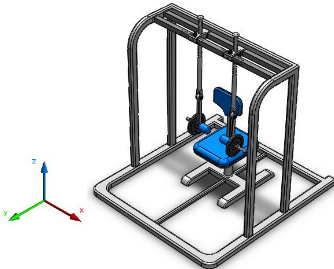
Slika 43. Naprava podešena za izvođenje pregibanja ili opružanja
