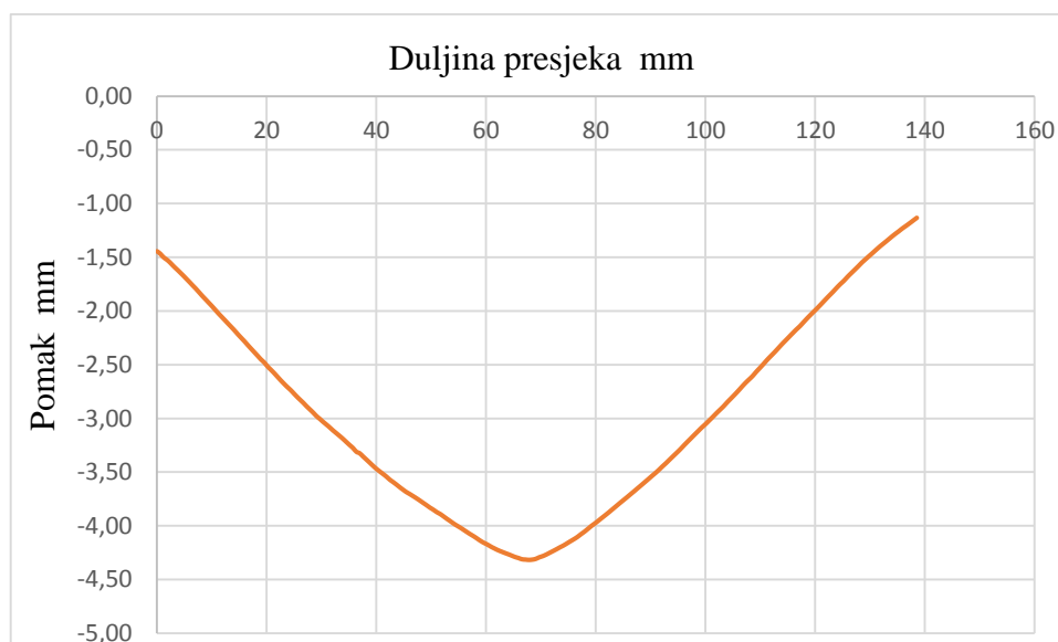
Slika 28. Dijagram pomak – duljina presjeka uzorka T_{12}
