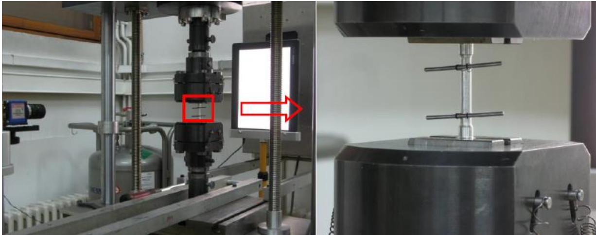
Slika 7. Mjerenje videoekstenzometrom [1]
