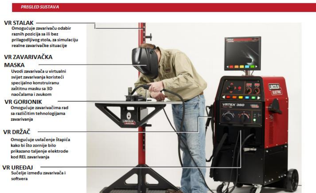
Slika 3.13. Lincoln Vrtex 360 [12].
