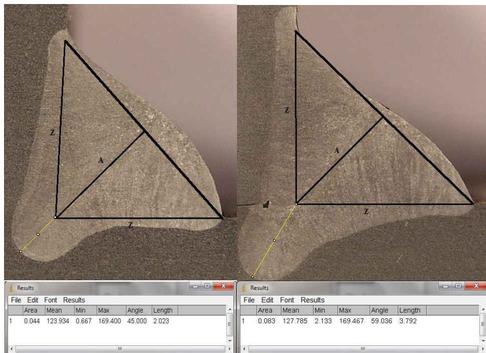
Slika 31. Prikaz mjerenja penetracije zavara. Uzorak „A“ - lijevo, uzorak „B“ - desno
