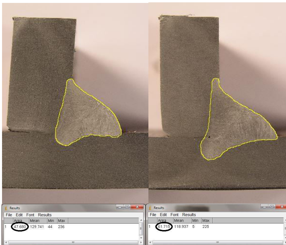
Slika 30. Prikaz mjerenja površine presjeka zavara. Uzorak „A“ - lijevo, uzorak „B“ - desno
