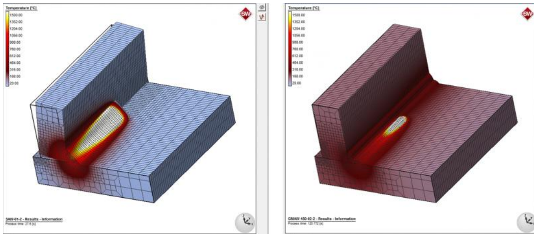
Slika 2. Prikaz deformacija u 'Simufact.welding-u' uslijed različitih procesa zavarivanja (lijevo bez, desno s predgrijavanjem) [4]
