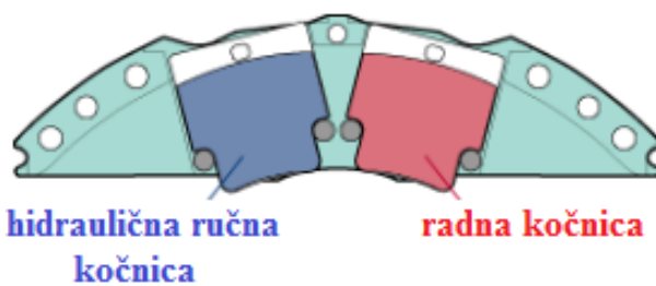
Slika 55 Četveroklipna kočiona kliješta D2
