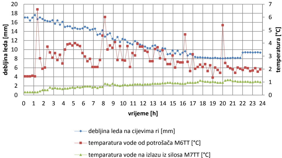
Slika 14. Topljenje leda u ovisnosti o temperaturi vode na ulazu i izlazu iz silosa
