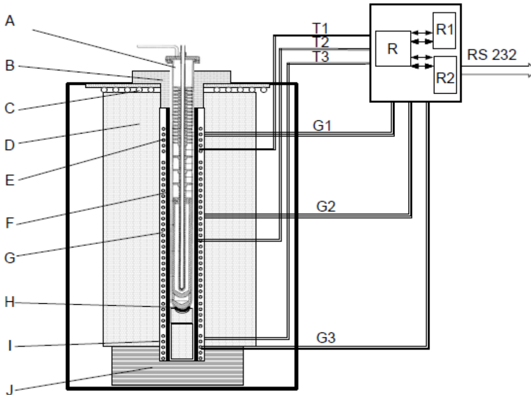
Slika 5. Presjek peći
