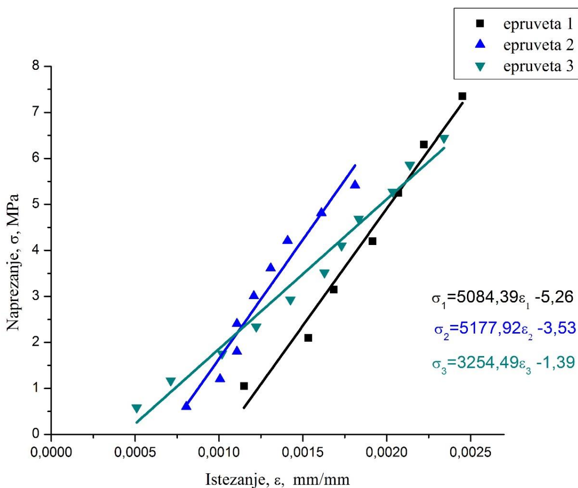
Slika 32. Dijagram naprežanje-istezanje Cellona epruveta (1, 2 i 3) slaganih u 15 slojeva
