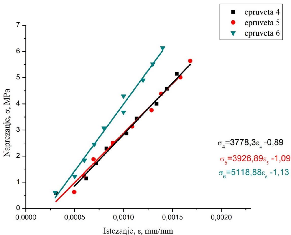
Slika 33. Dijagram naprežanje-istežanje Cellona epruveta (4, 5 i 6) slaganih u 15 slojeva
