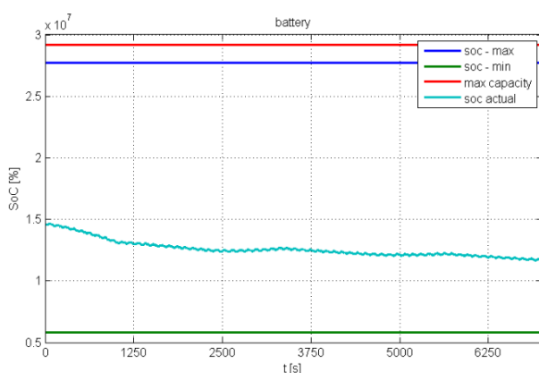
Slika 17. Ponašanje baterije čiji je kapacitet jednak trećini početnog kapaciteta
