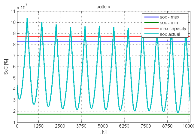
Slika 28. Ponašanje baterije zadanih karakteristika za postrojenje od 4 serijske i 37 paralelnih jedinica
